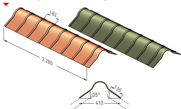
cumbrera polivalente de HSP y de Ecotres
