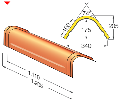
cumbrera multished en polimglass
