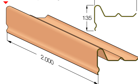
unión para frontalino en polimglass
