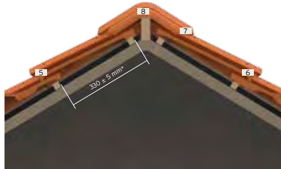
Cumbrera
